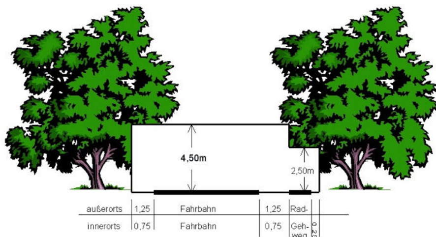
Lichtraumprofil
