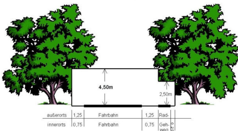
Lichtraumprofil
