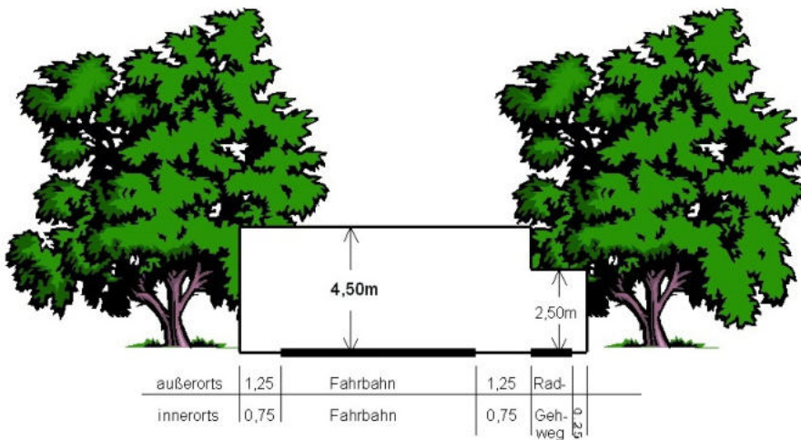
Lichtraumprofil
