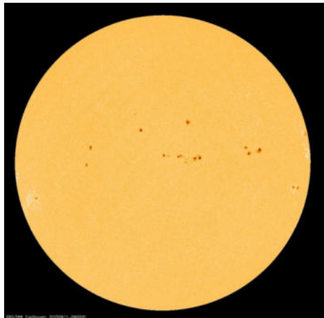
Sonne im Weißlicht am 11.08.2025 vom HMI Image
