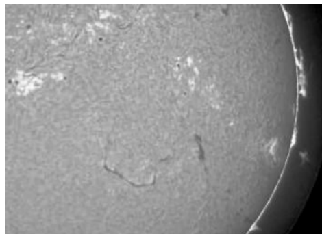
Sonne im Wasserstoff-Licht am 11.08.2025 von PIC Teide
